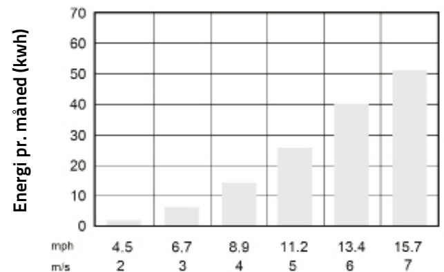
Årlig gennemsnit vind hastighed
