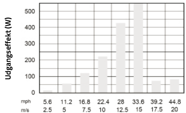
Kontinuerlig vind hastighed
